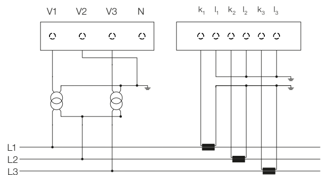
Medição com 2 TPs e 3 TCs
